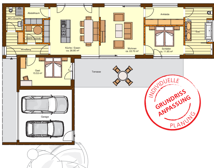
Grundriss
