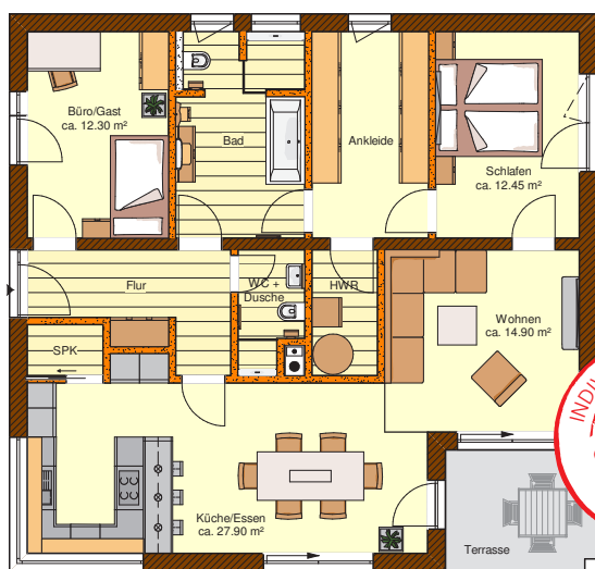
Grundriss
